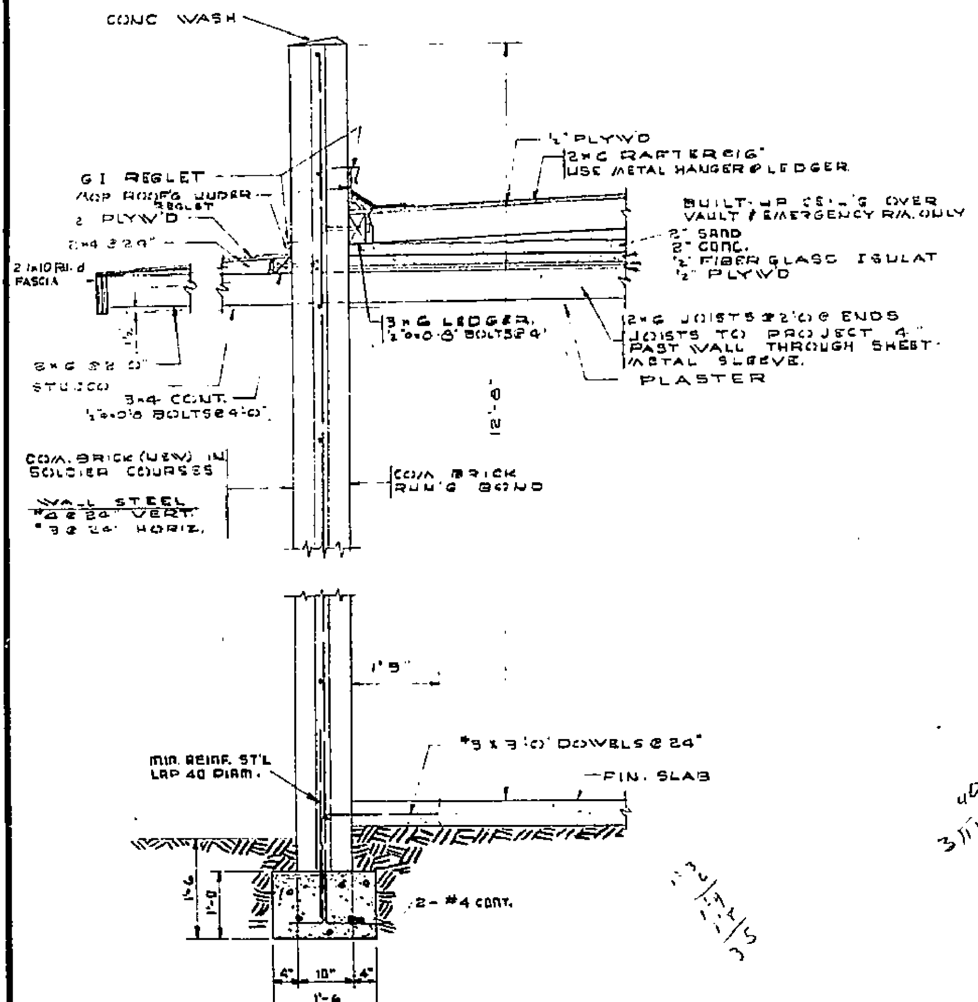
SECTION B SCALE: 3/4"=1'-0"
