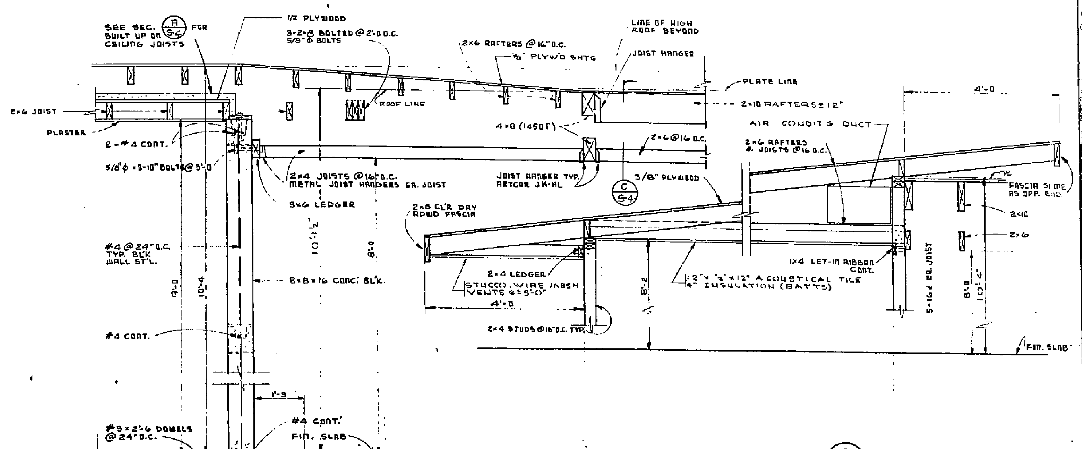
SECTION C SCALE: 3/4"=1'-0"
