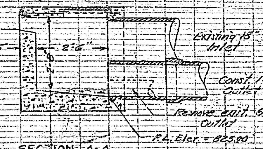
SECTION A-A Scale: 1 in. = 2 ft.
