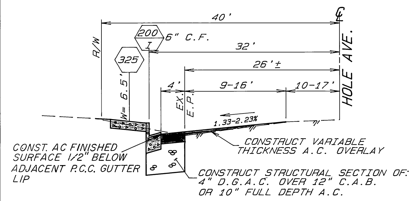
TYP. SECT. HOLE AVE. STA. 29+50 TO 31+45 SCALE: HORIZ. 1" = 10' VERT. 1" = 2'
